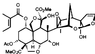
(1) Azadirachtin
